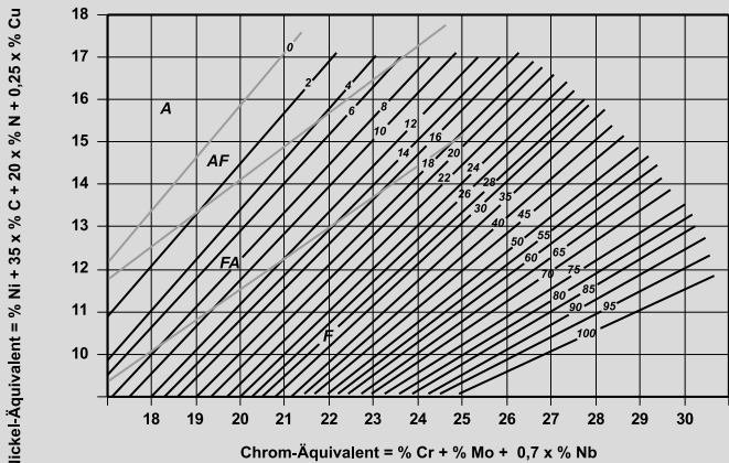
WRC - 92 - Diagramm
