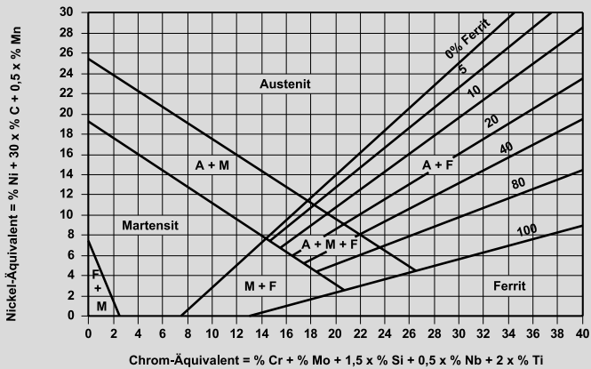
Schaeffler - Diagramm (nach A. L. Schaeffler, Metal Progress Nov. 1949, Seite 680 bis 680-B)
