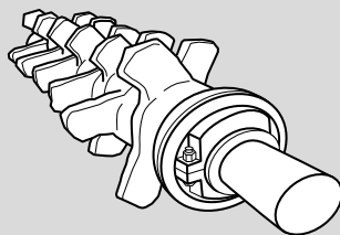
Sinterbrecher
