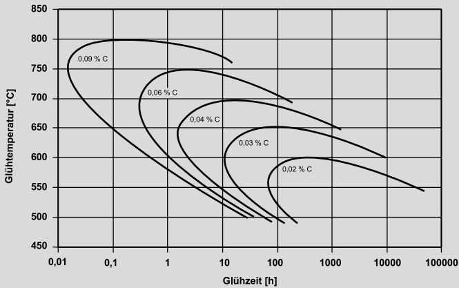
Kornerfallbereiche für 18/8-Chrom-Nickel-Stähle in Abhängigkeit vom gelösten Kohlenstoffgehalt (nach H.J. Rocha)
