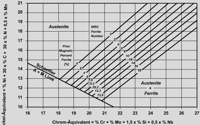
DeLong - Diagramm
